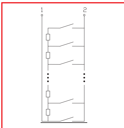
Wiring diagramm
